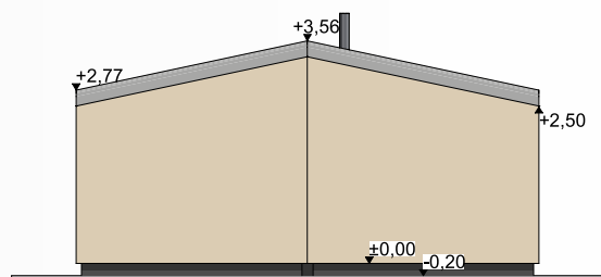
ELEWACJA TYLNA
