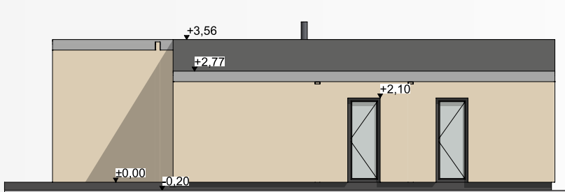
ELEWACJA PRAWA
