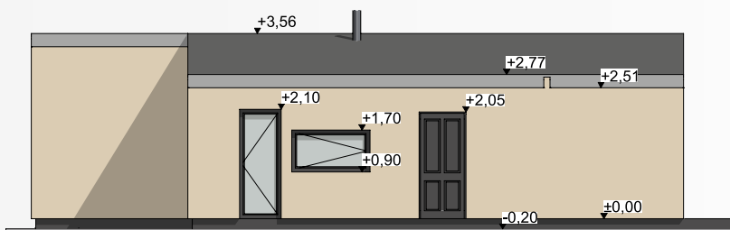
ELEWACJA LEWA
