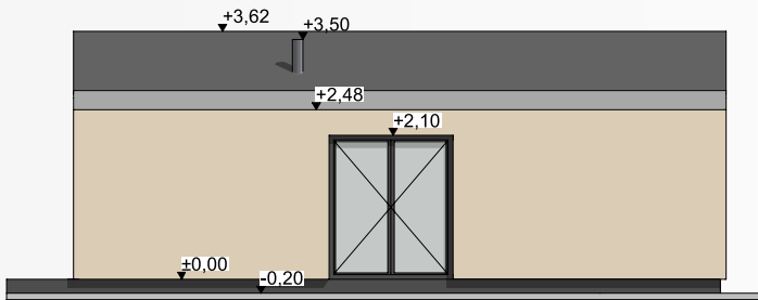
ELEWACJA PRAWA
