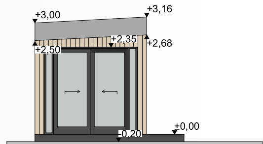
ELEWACJA LEWA
