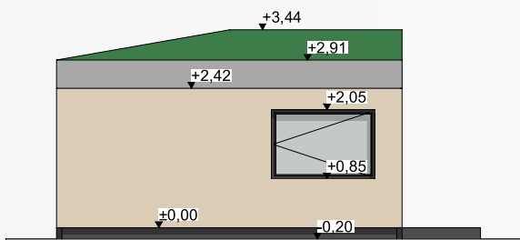
ELEWACJA LEWA
