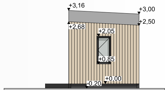
ELEWACJA PRAWA
