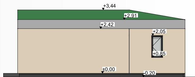
ELEWACJA TYLNA
