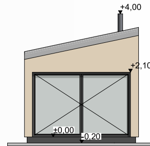
ELEWACJA FRONTOWA
