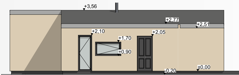
ELEWACJA LEWA
