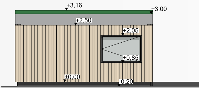
ELEWACJA TYLNA
