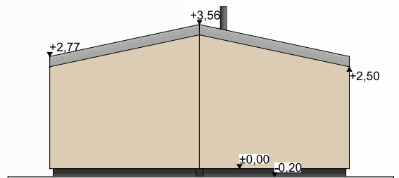
ELEWACJA TYLNA
