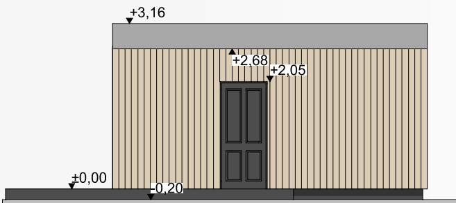
ELEWACJA FRONTOWA
