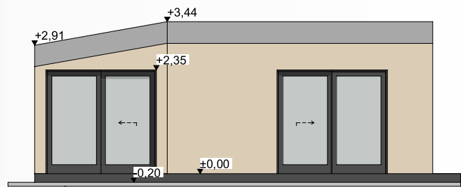
ELEWACJA FRONTOWA
