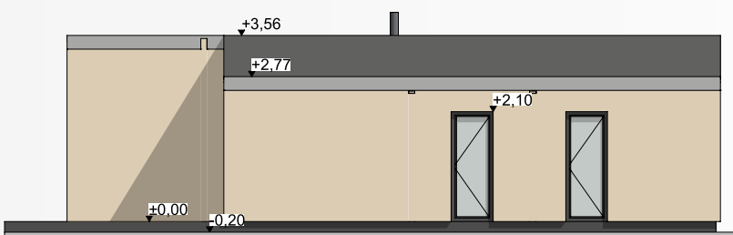
ELEWACJA PRAWA
